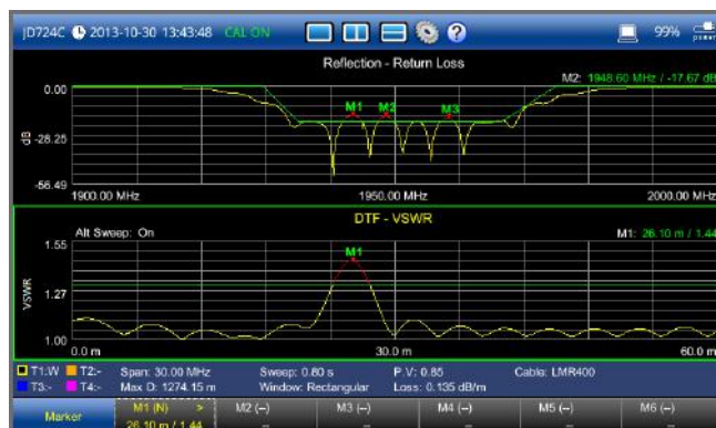
Balayage alternatif en mode DTF
