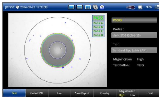
Inspection des fibres optiques
